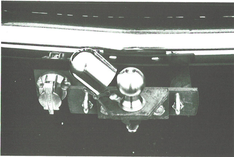
Crochet d'attelage avec faisceau électrique.
