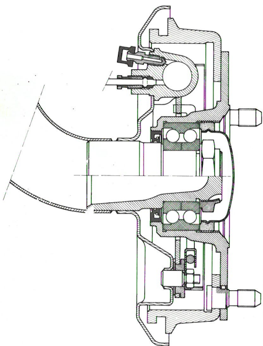
SCHNITT DURCH DIE NABE
