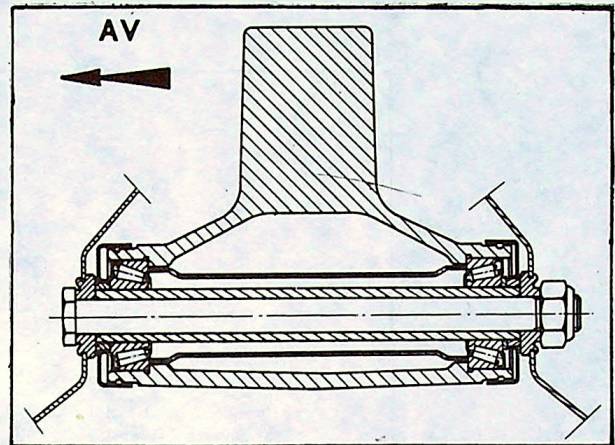
BRAS SUPÉRIEUR
