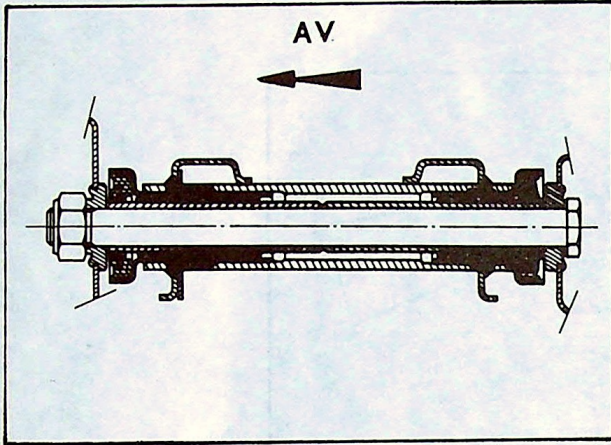
BRAS INFÉRIEUR
